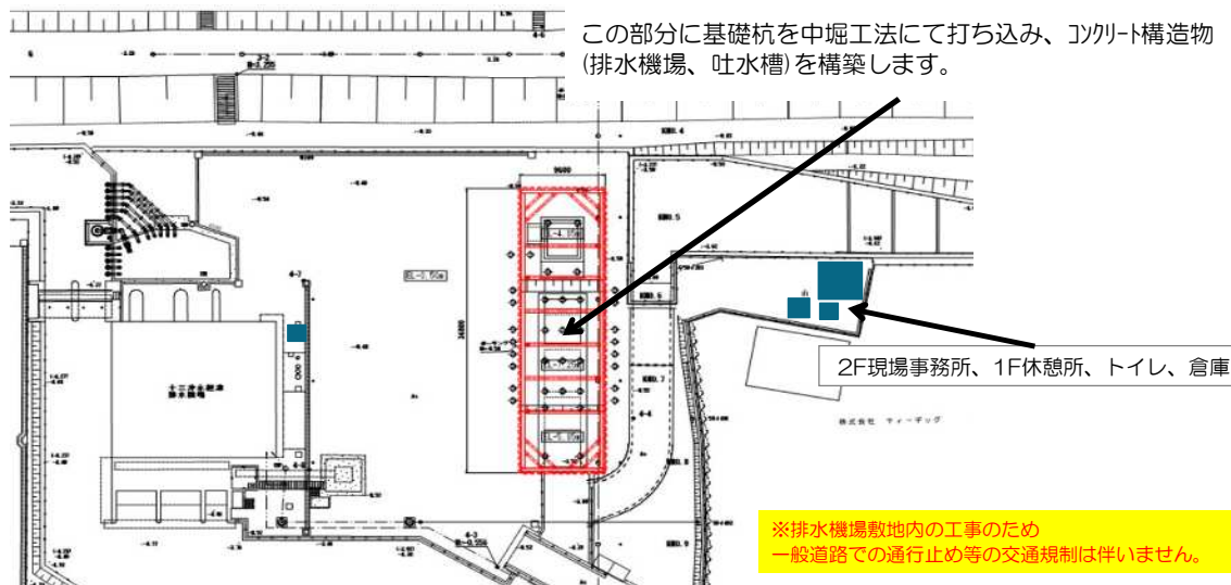
工事詳細平面図
